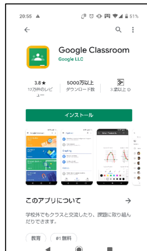
Android での例→
